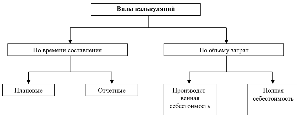
Рис. 29. Группировка калькуляций
