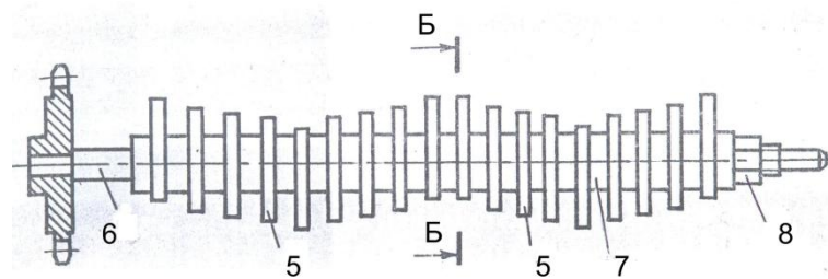
Рис.4 - Заборный орган в сборе
