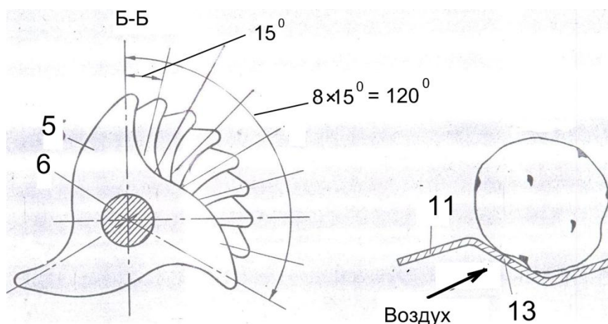
Рис.5 - Сечение Б-Б на рис.4 и вариант нахождения клубней на клин
