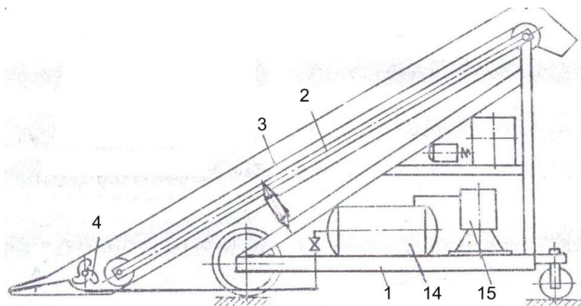
Рис. 1 - Самоходный автокар для погрузки навалочных грузов (общий вид)
