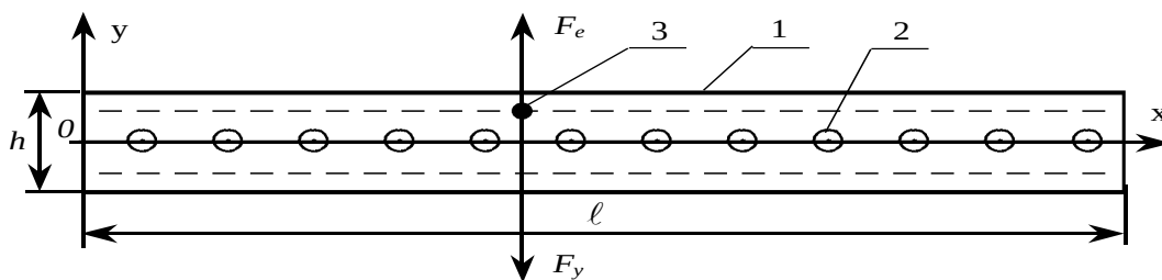
Рис. 2 - Схема силового взаимодействия в сепараторе УМС
