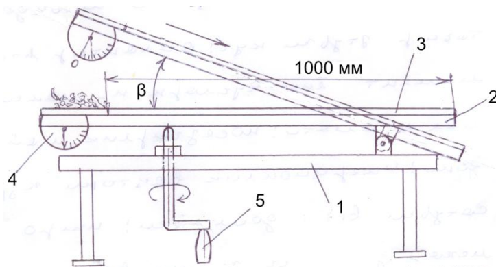
Рис. 2 - Опытный прибор скольжения
