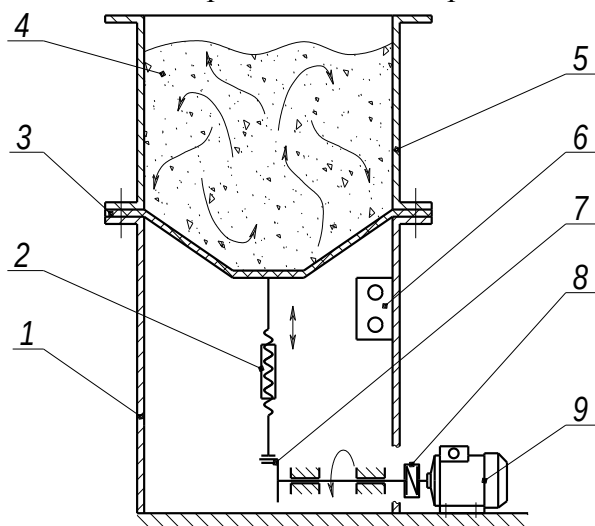
Рис. 1 - Принципиальная схема установки для создания виброкипящего слоя зернового материала:
