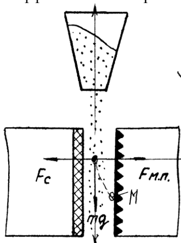
Рис. 1- Схема силового взаимодействия в сепараторах УСС
