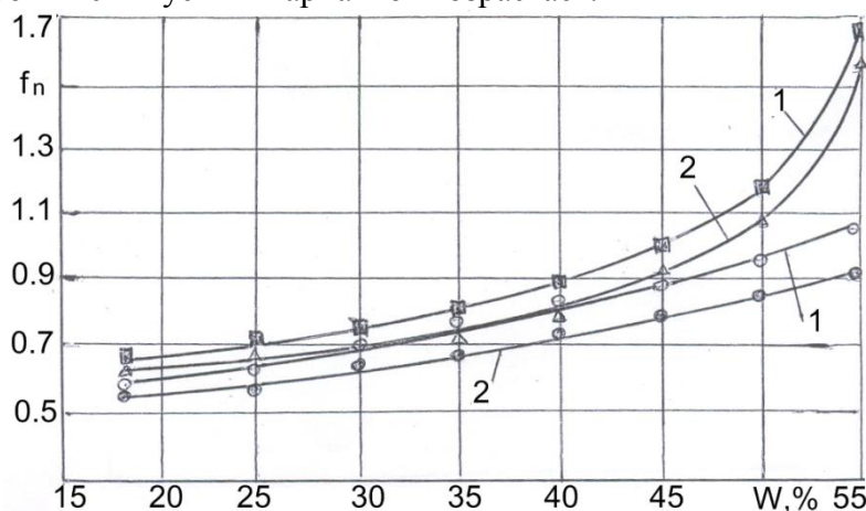
Рис. 3 - График изменения коэффициента трения покоя ( f_n ) в зависимости от влажности подвяленного винограда ( W ).
