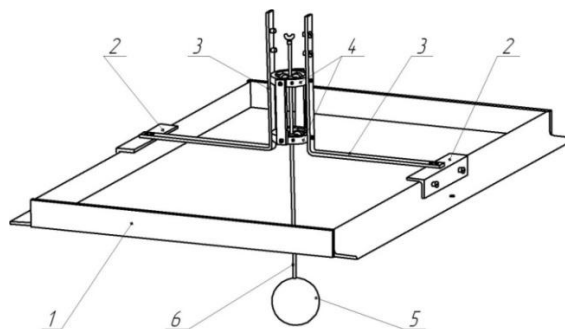
Рис. 2 - Приспособление для измерения подъемной силы:
