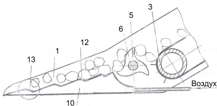
Рис.3 - Разрез А-А на рис.2
