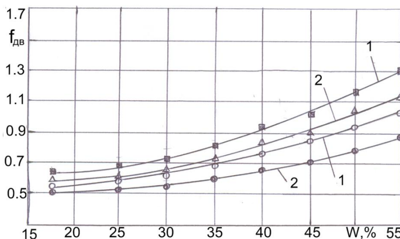
Рис. 4 - График изменения коэффициента трения движения ( f_{дв} ) в зависимости от влажности продукта (W)
