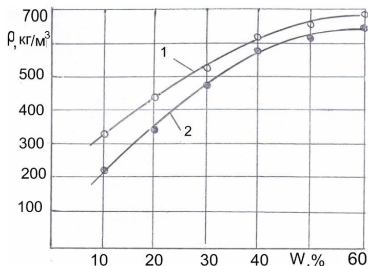
Рис. 1 - Зависимость насыпной плотности ( \rho ) подвяленного винограда от его влажности ( W )
