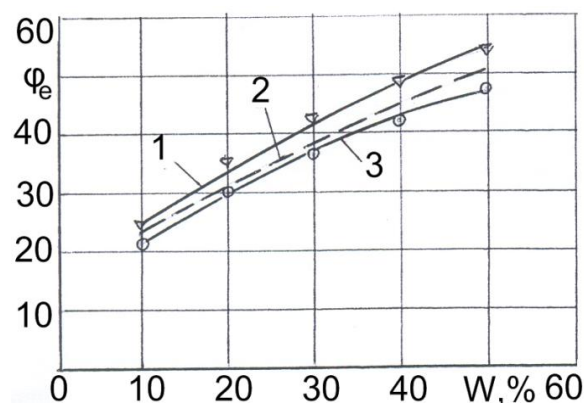
Рис. 5 - Изменение угла естественного откоса массы подвяленного винограда ( \varphi_e ) в зависимости от их влажности (W):
