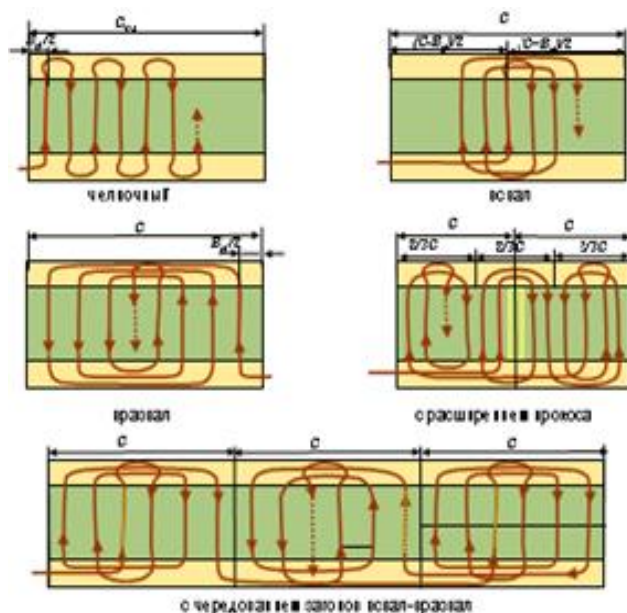
Рис. 3.5 Способы движения пахотных МТА
