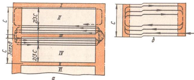
Рис. 3.15 Способы движения зерноуборочных комбайнов а - гоновый с расширением прокосов; б - гоновый по ходу часовой стрелки; I— обкос боковой; II, IV и VI— первый, второй и третий загоны; III и V— прокосы; C— ширина загона.
