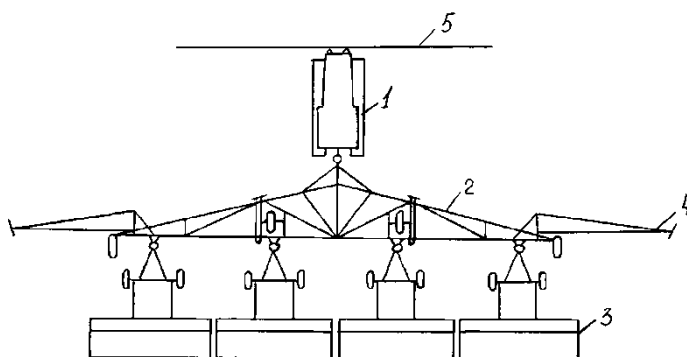
Рис. 1.15 Схема четырехсечального посевного агрегата Т-4А + СП-16А + 4СЗП-3,6:
