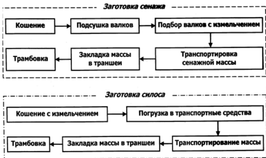
Рис.3.18. Технологические схемы заготовки сочных кормов
