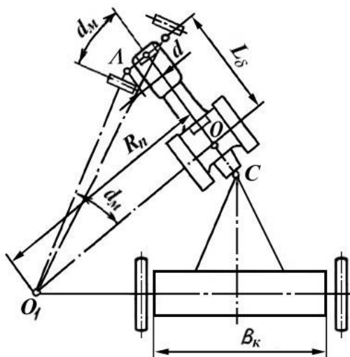
Рис. 1.18 Схема для определения радиуса поворота агрегата
