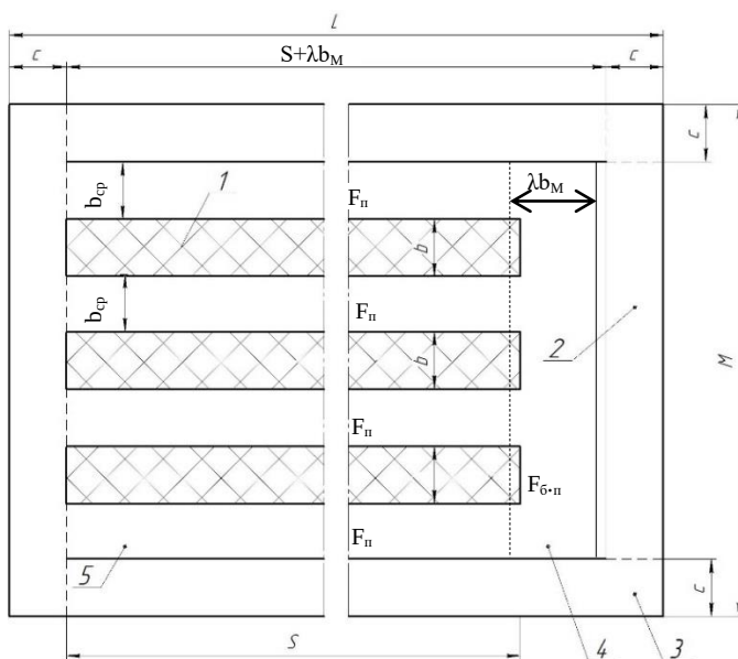
Рис. 4.20 Схема к расчету площади зоны хранения машин на открытых площадках
