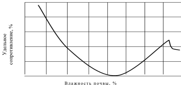
Рис. 1.6 Характер изменения удельного сопротивления плуга в зависимости от влажности почвы
