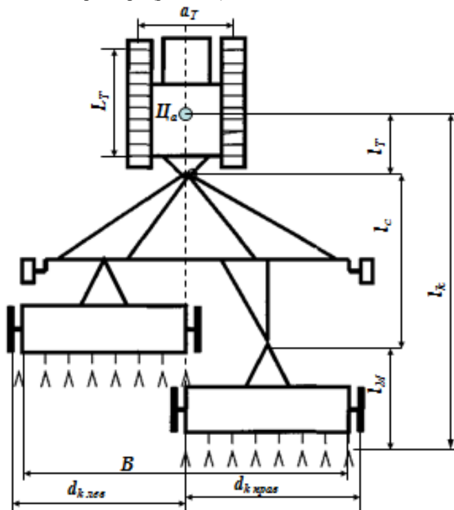
Рис.1.16 Кинематические характеристики агрегата
