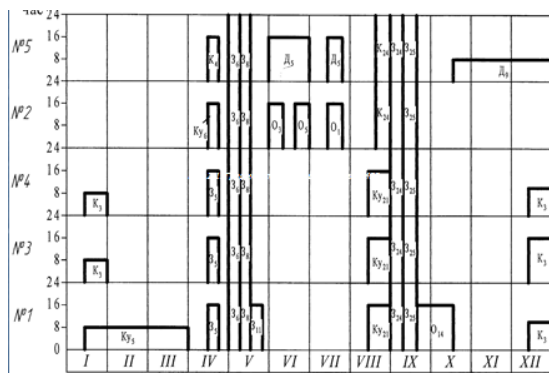
Рис. 3. 22 График потребности в тракторах К-730М
