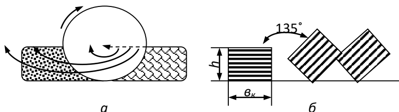
Рис. 1.. Технологические процессы при дисковании вспашке почвы: а – дискование; б – вспашка
