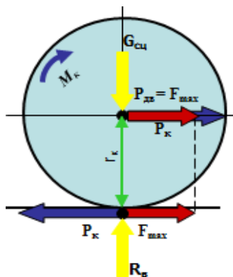
Рис.1.11 Схема образования движущей силы при недостаточном сцеплении движителей трактора с почвой
