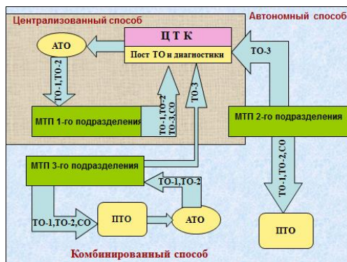
Рис. 4.18 Методы организации ТО машин
