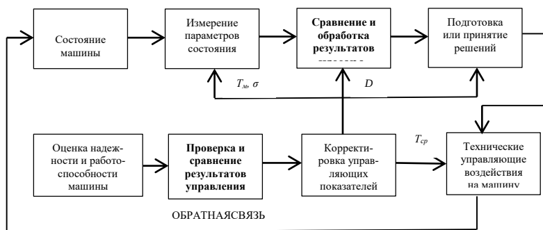
Рис. 2.2 Схема управления техническим состоянием машины
