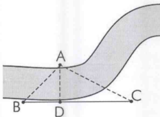
Определение ширины реки способом засечек с опусканием
